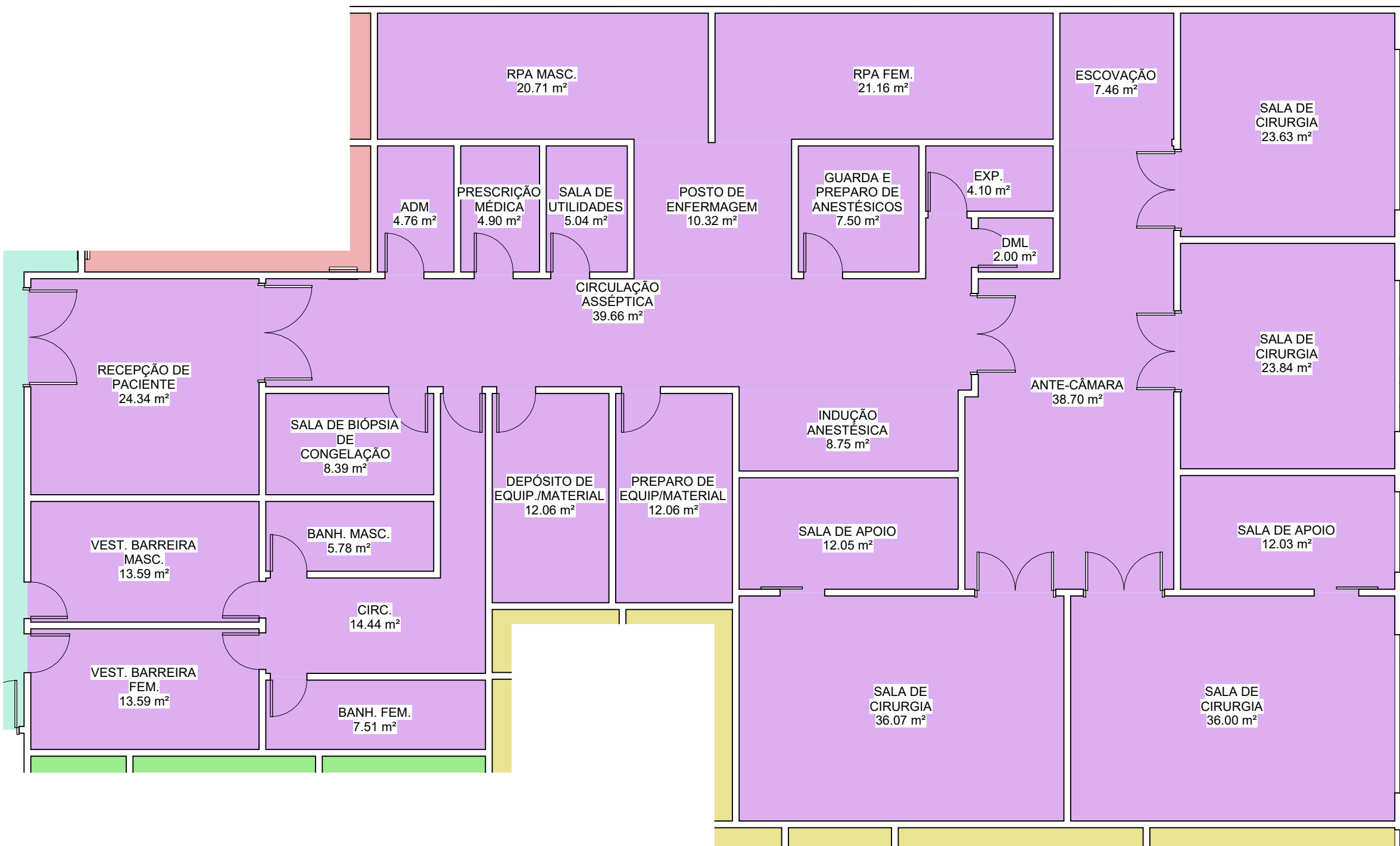
1 Térreo - CC 1 : 100
