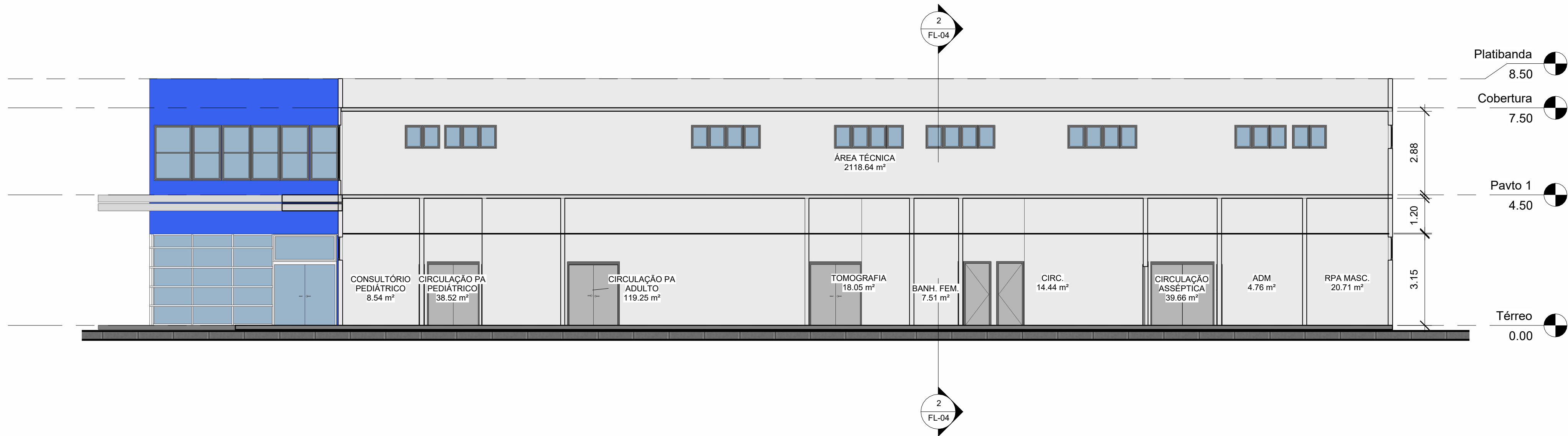
1 Corte 1 1 : 100
