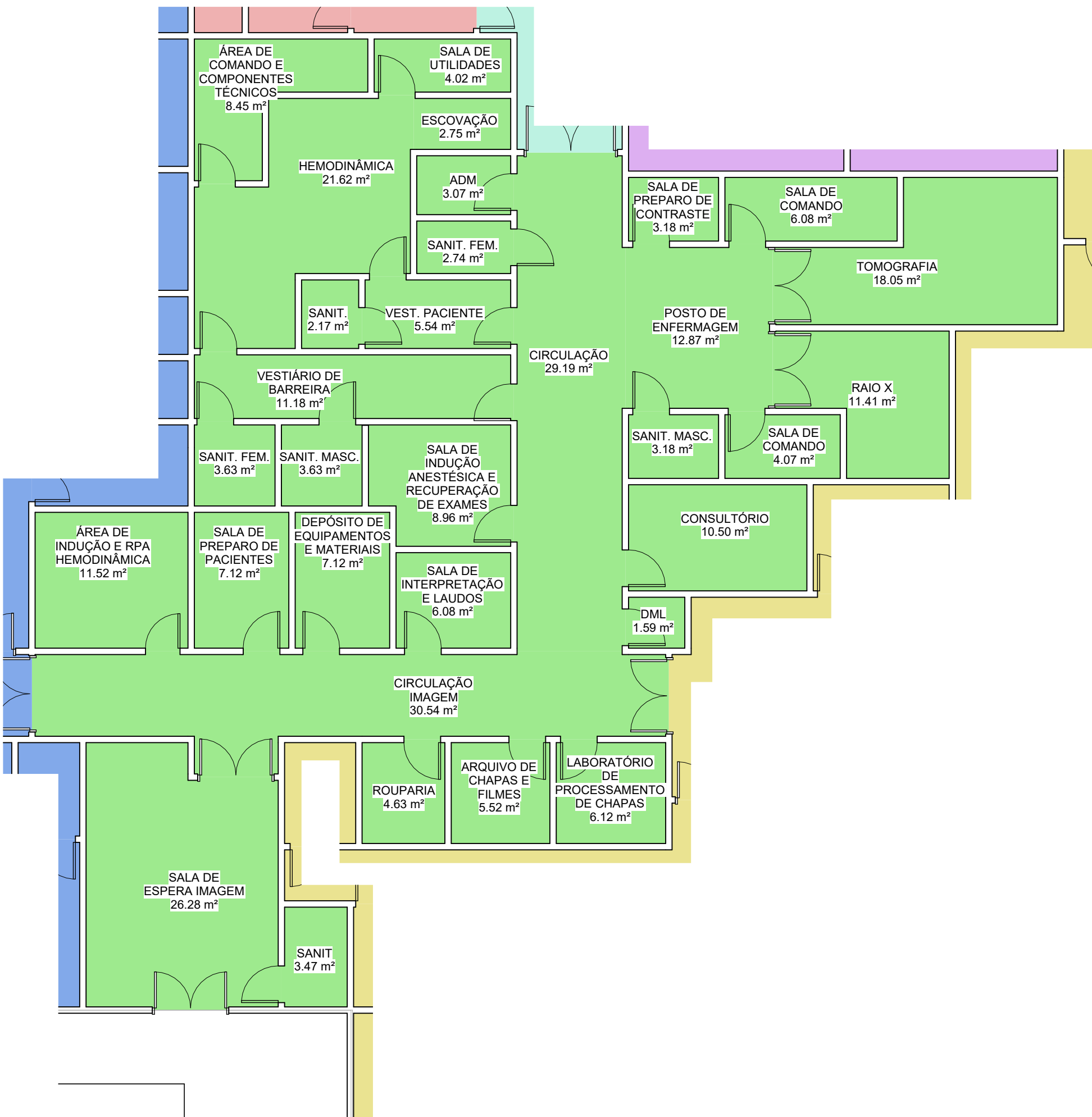
2 Térreo - IMAGEM 1 : 100
